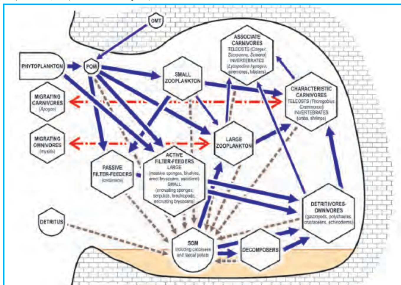
Fig. 6.1. Modèle théorique de la structure et du fonctionnement de l'écosystème des grottes marines de la Méditerranée. Les biocénoses des grottes semi-obscurées et sombres sont indiquées pour chaque composante de l'écosystème (dans des encadrés). Les flèches noires indiquent l'intensité des flux de matière organique, les principaux flux étant représentés par des flèches noires pleines. Les flèches verticales en pointillés représentent la matière organique qui atteint le fond de la grotte, telle que la matière organique d'origine terrestre (OMT), la matière organique particulaire en suspension (POM), les boulettes fécales et les carcasses d'organismes morts. Les flèches horizontales en pointillés indiquent les principaux apports de matière organique dans les grottes, soit par advection due au mouvement de l'eau (pour les POM et les détritus), soit par la migration horizontale nycthémerale des mysidacés et du poisson cardinal Apogon imberbis. D'après Rastorgueff et al. (2015a).
