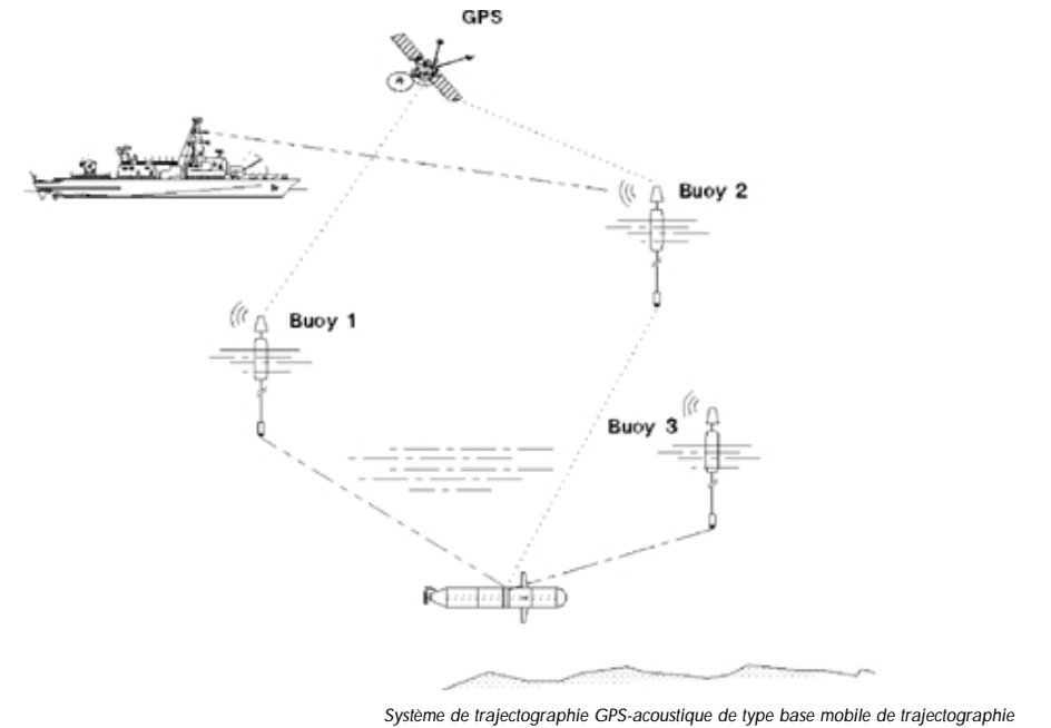
Système de trajectographie GPS-acoustique de type base mobile de trajectographie
